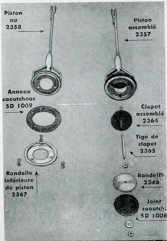
Robinet-soupape tout acier F. S. A
